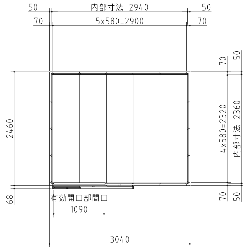
平面図
